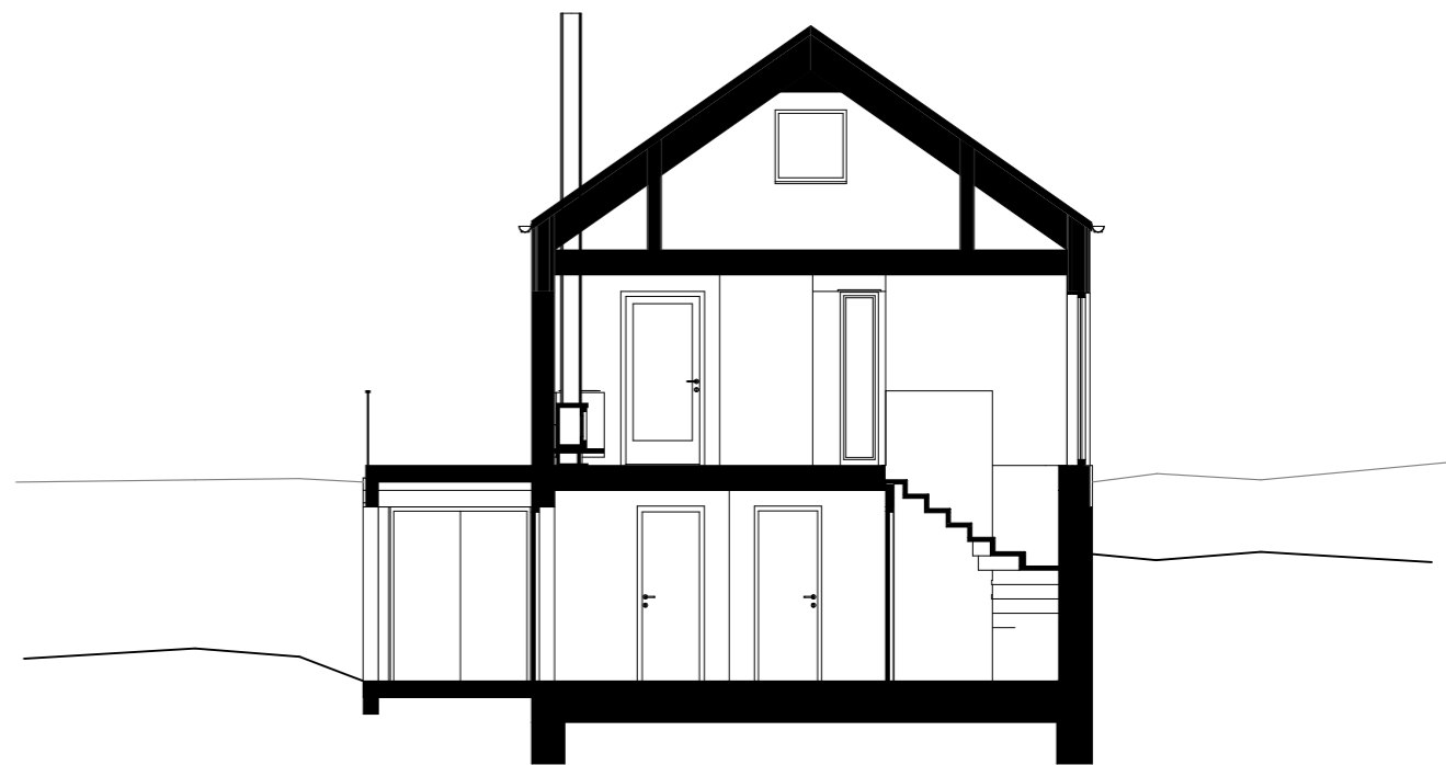
TVERRSNITT AA
