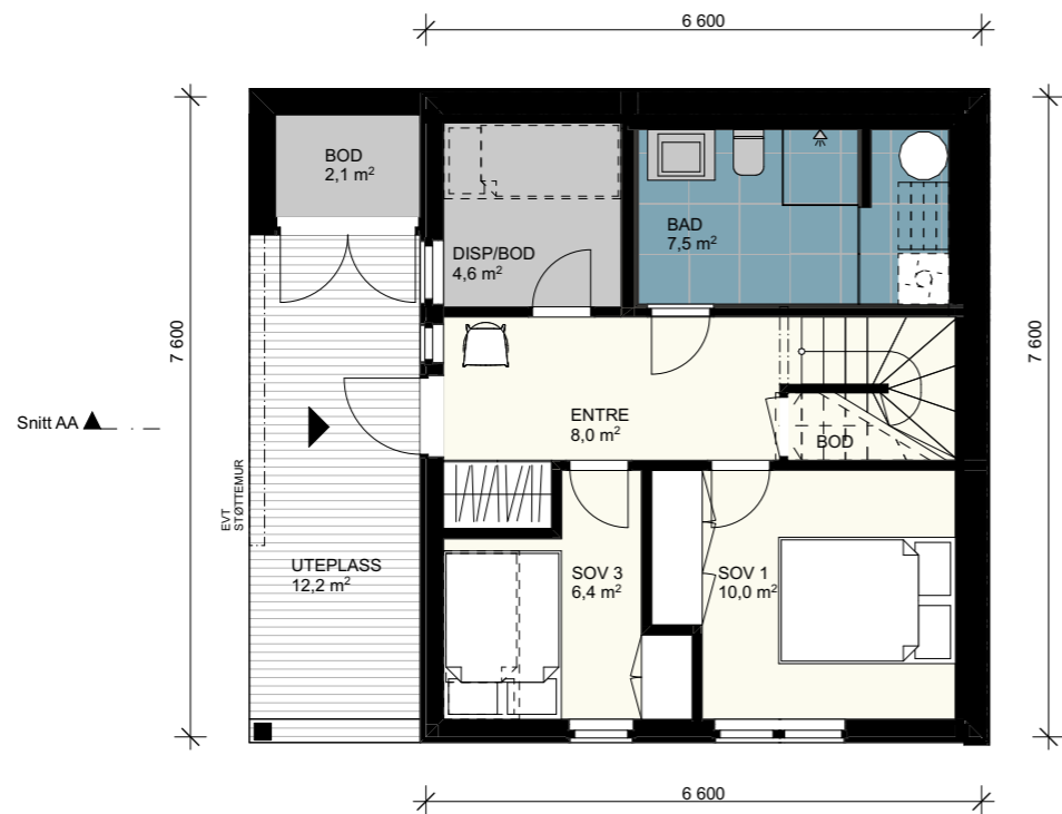
PLAN 1. ETASJE
