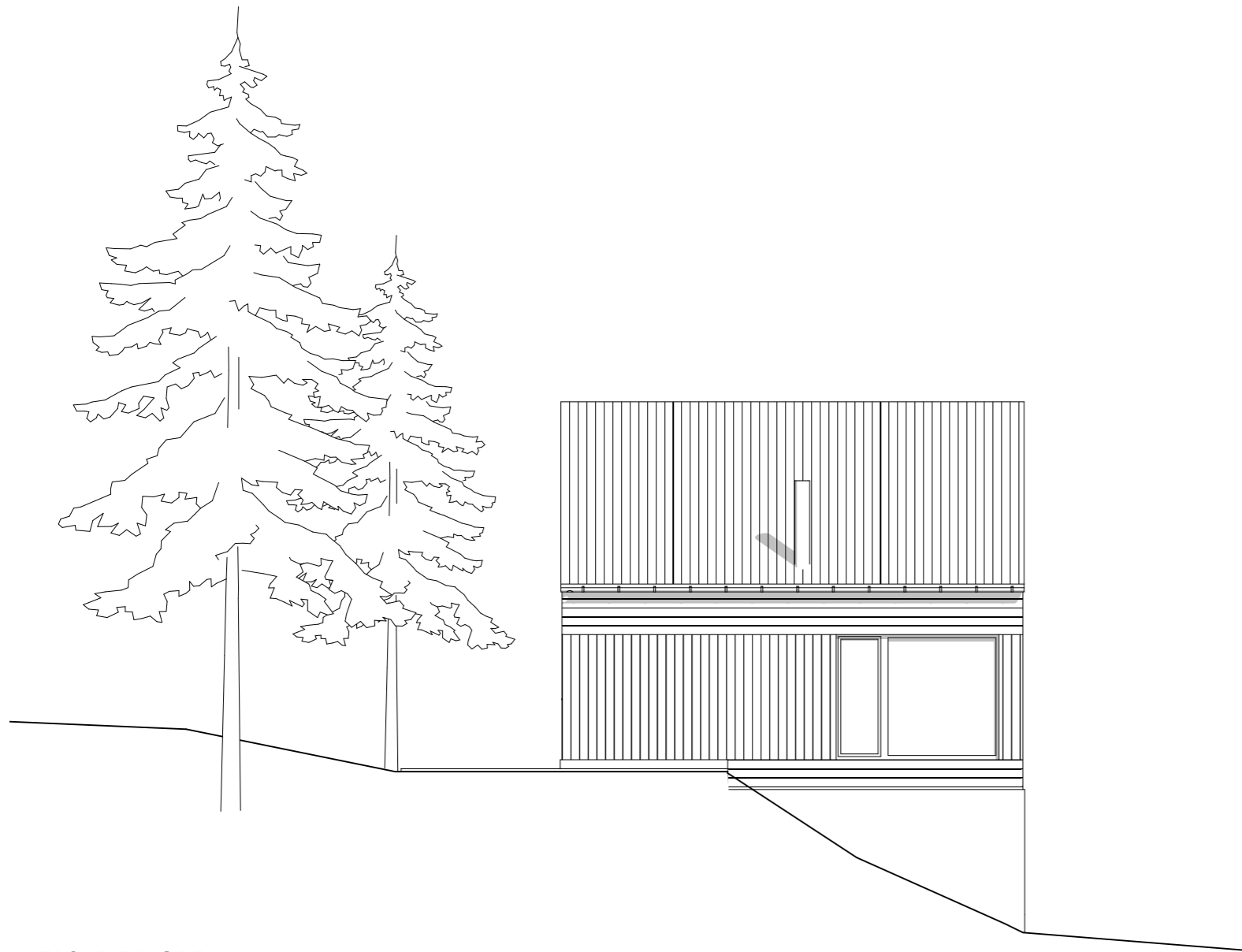
FASADE NORD
