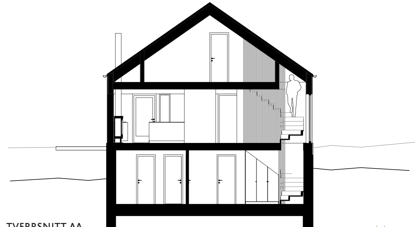
TVERRSNITT AA
