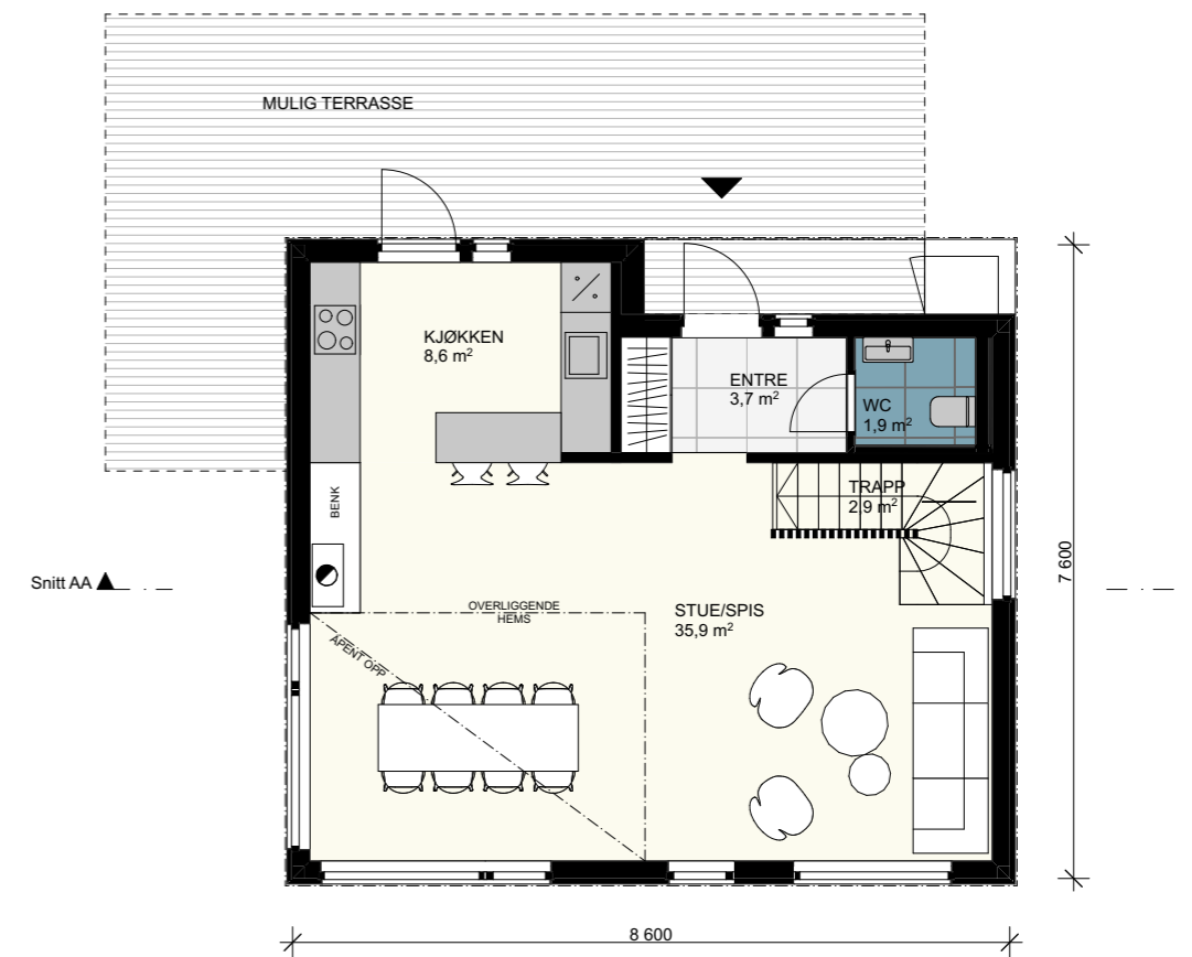
PLAN 2. ETASJE
