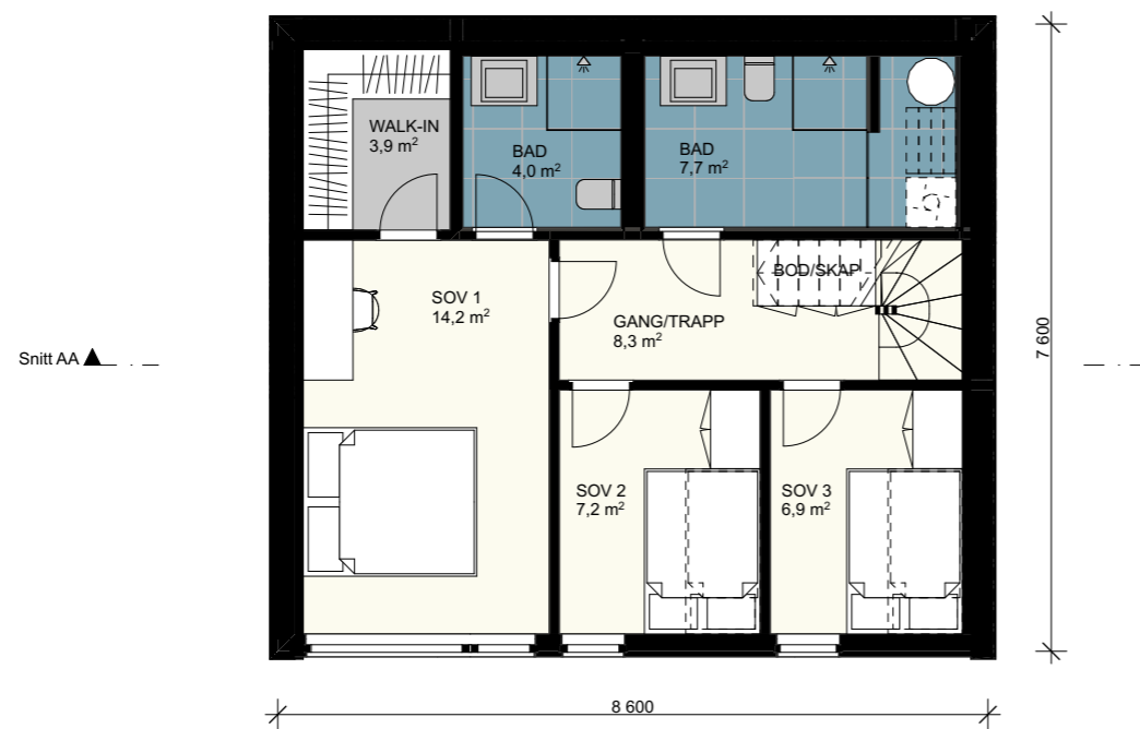
PLAN 1. ETASJE
