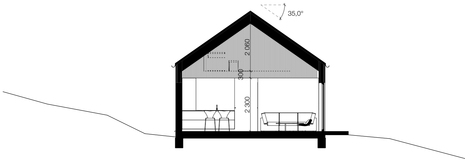
TVERRSNITT
