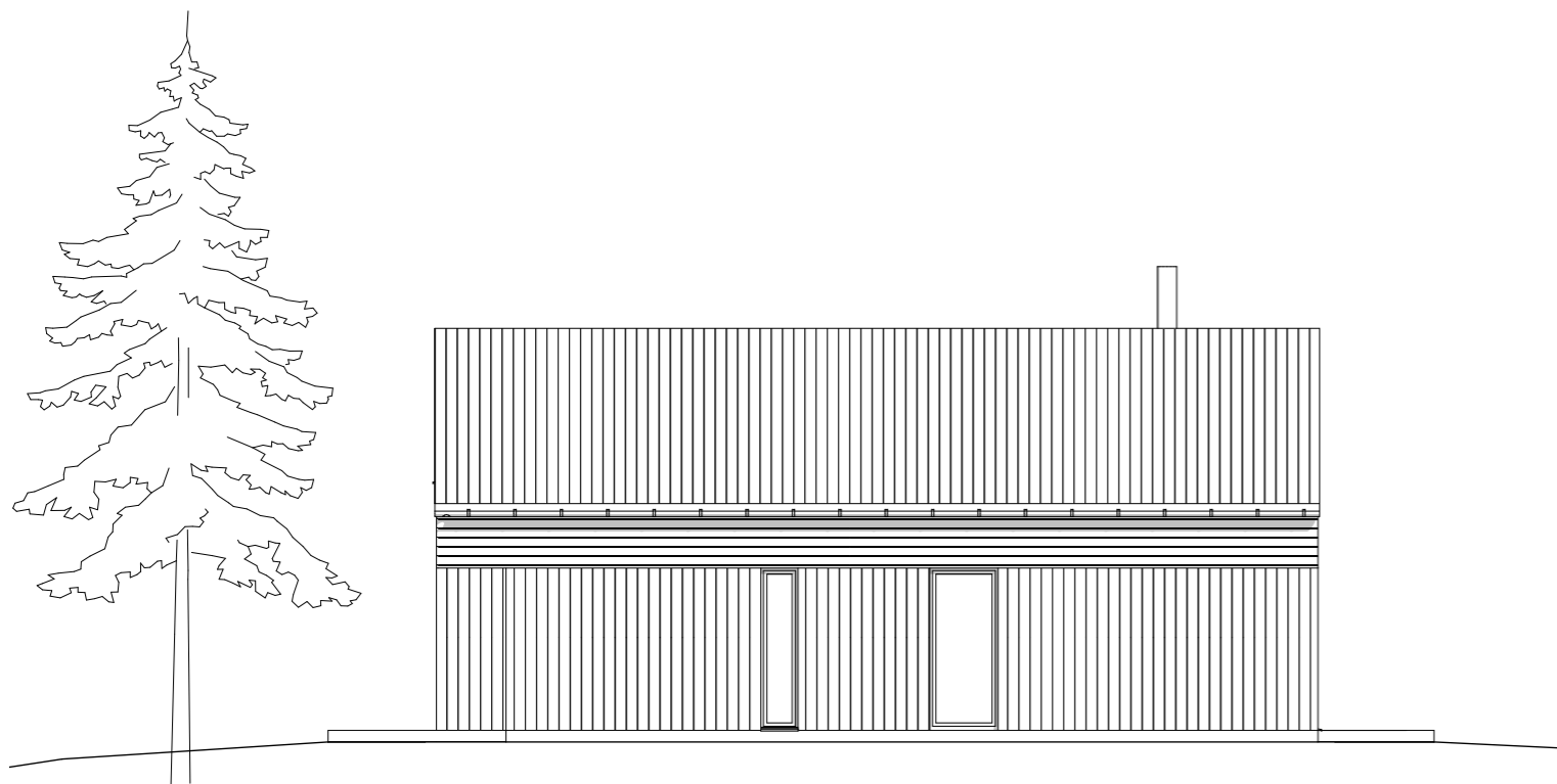
FASADE SØRVEST
