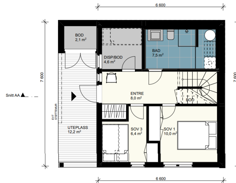
PLAN 1. ETASJE
