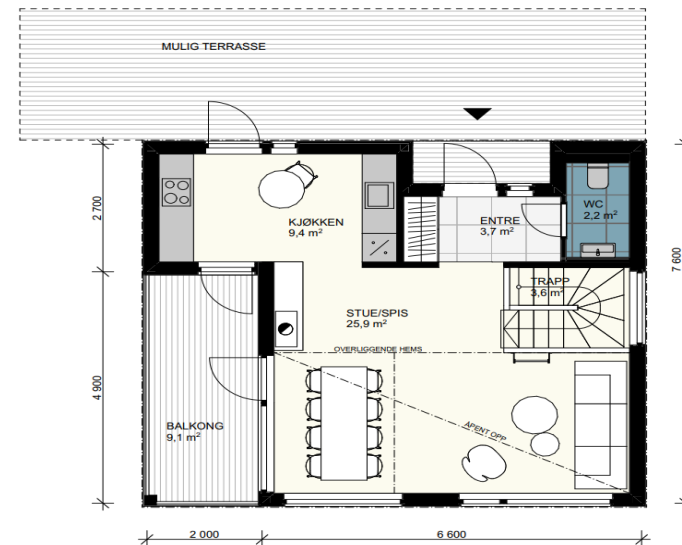
PLAN 2. ETASJE
