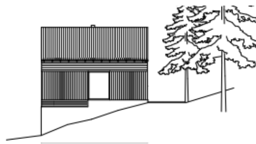
FASADE SØR
