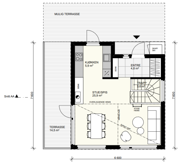
PLAN 2. ETASJE
