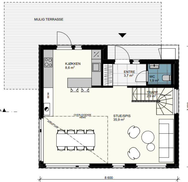
PLAN 2. ETASJE
